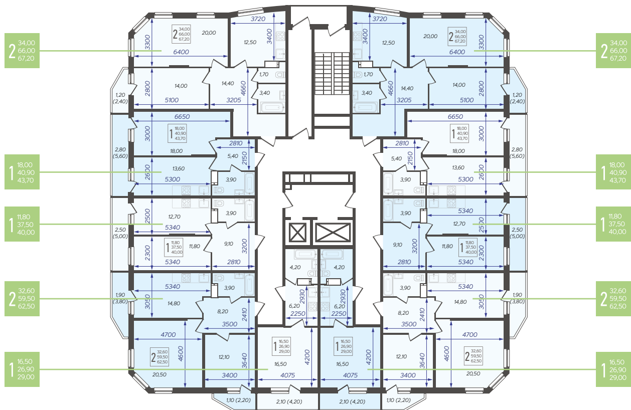
ЭТАЖ 2-3
